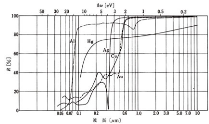
いろいろな金属の反射率
