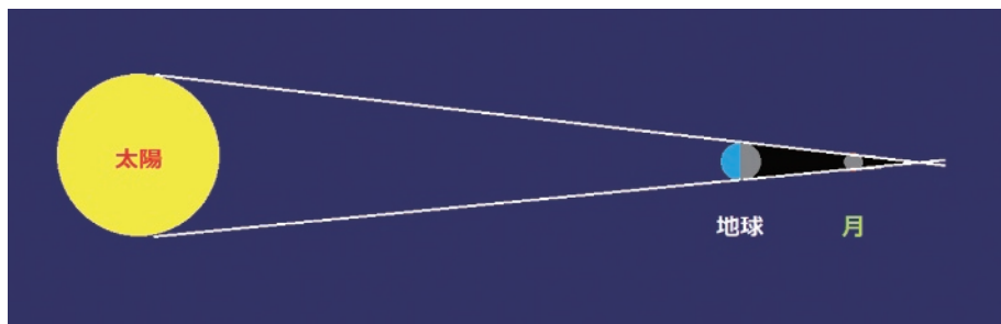
月食の仕組み: 月が地球のかげに入るのが月食
