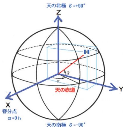
図2. 赤道座標系の直交座標
