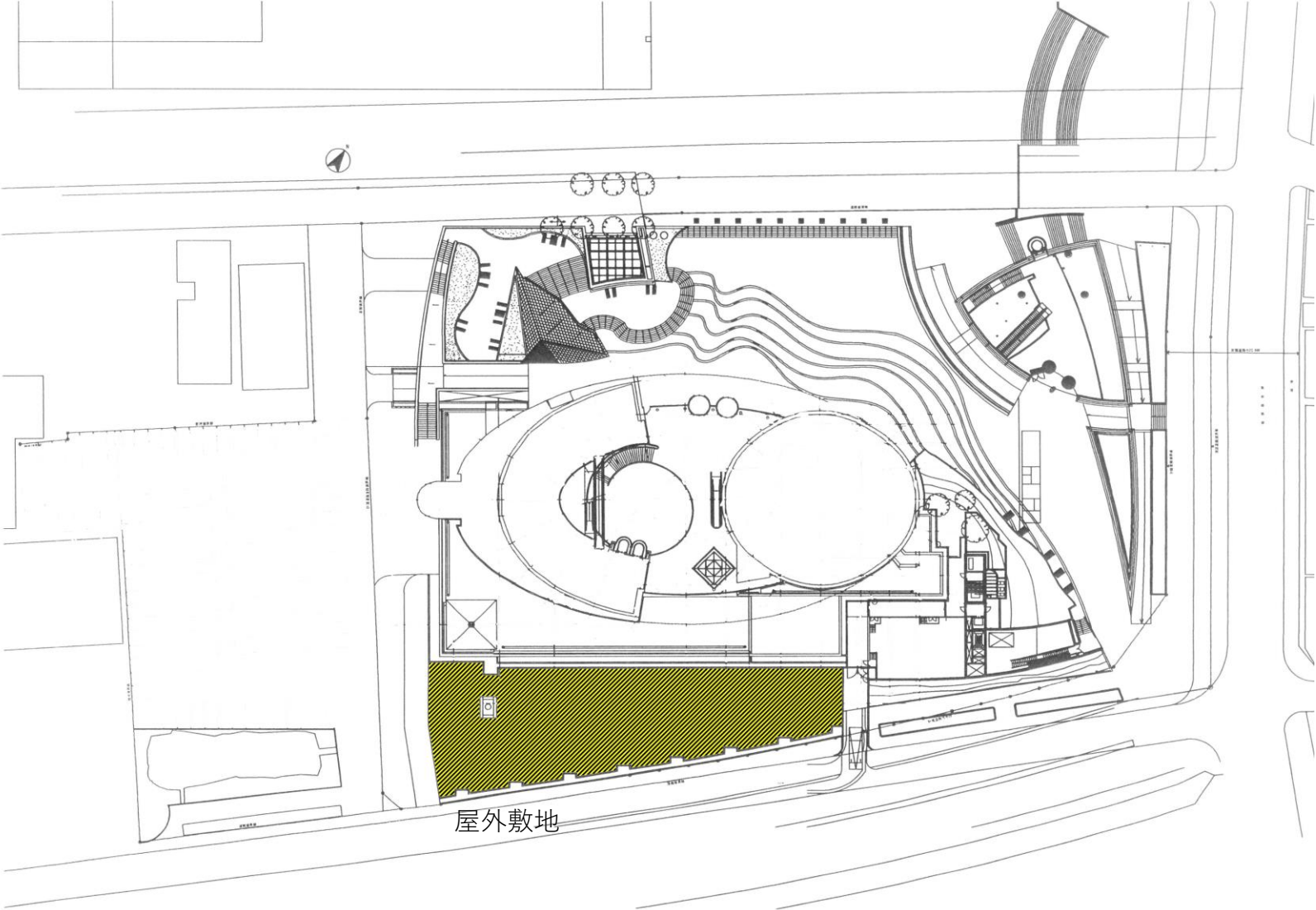
参考图6 (敷地)
