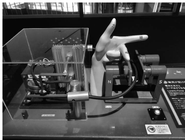
写真1.法則展示「電流が受ける力」
