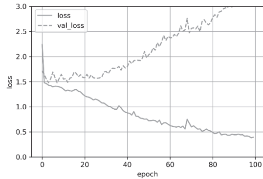
図 9 損失関数の変化(解析雨量データを追加)
