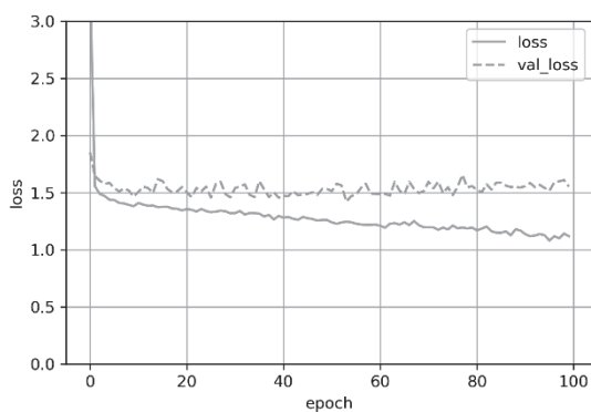
図 7 損失関数の変化(雲画像のみで学習)
