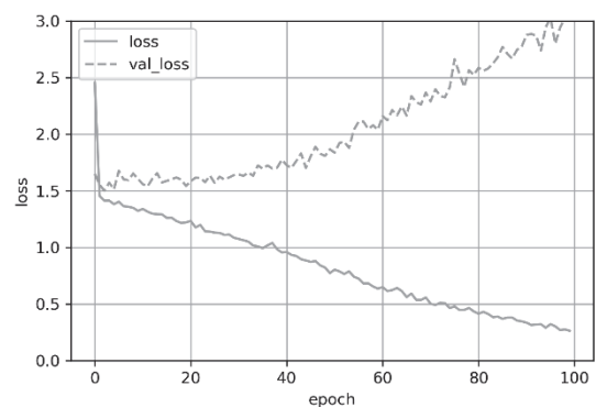
図 9 損失関数の変化(アメダス観測値データを追加)
