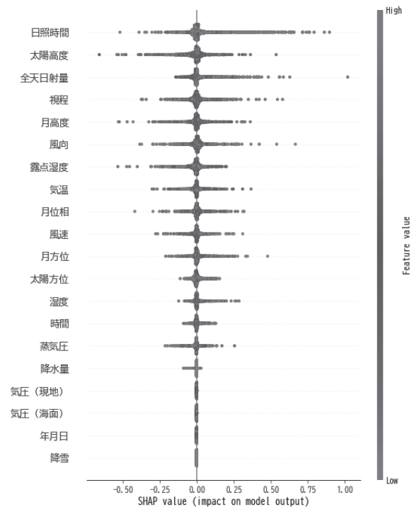
図 11 SHAP 値による分析
