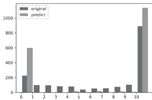
図 8 雲量の分類(雲画像のみで学習)
